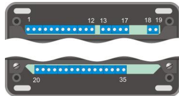
Рисунок 6.3 Клеммы БПС 24В.
