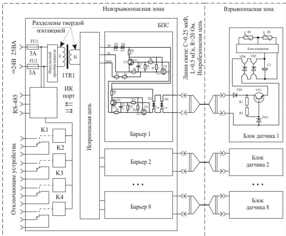
Рисунок 5.2 Средства обеспечения взрывозащищенности БПС 24В
